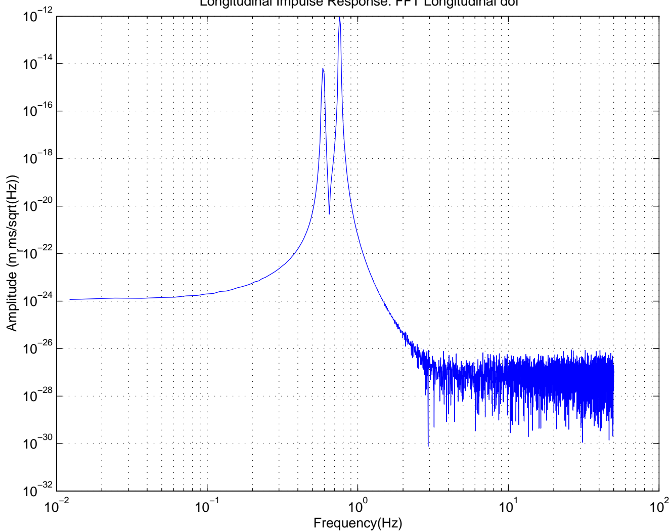
Longitudinal Impulse Response: FFT Longitudinal dof
