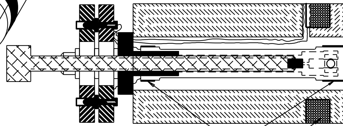
TYP. (6) (5) SECTION A-A SCALE 2:1
